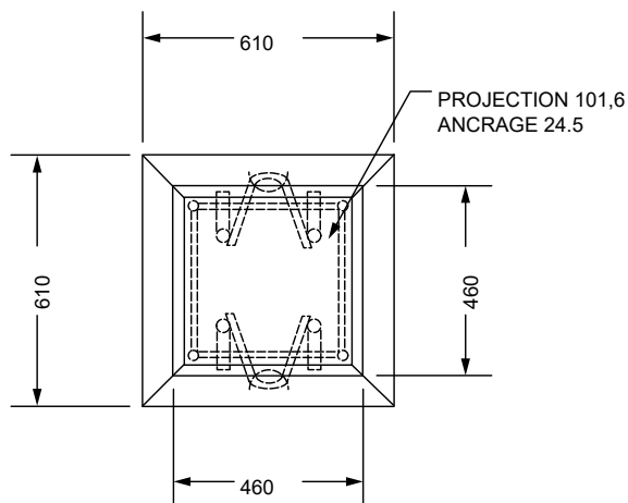
VUE DESSUS
