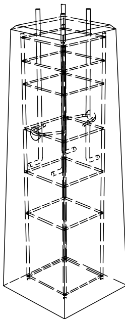
VUE ISOMETRIQUE
